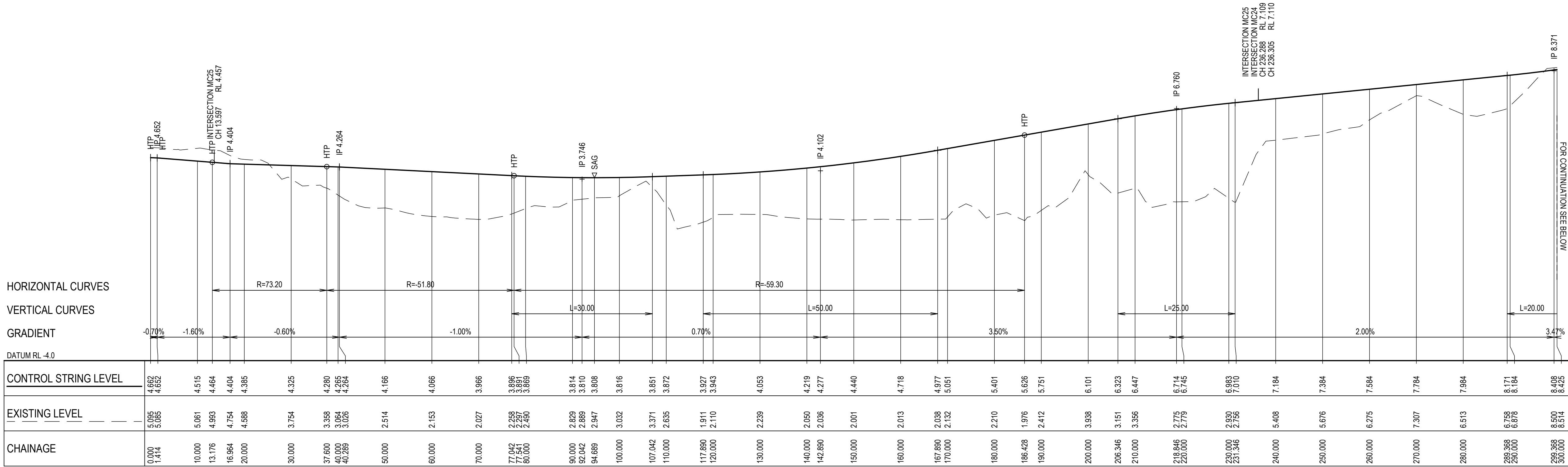
MC03 LONGITUDINAL SECTION SCALE 1:500 HORI. 1:100 VERT.
