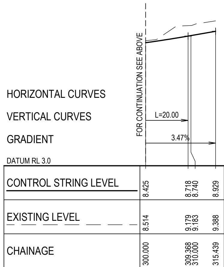
MC03 LONGITUDINAL SECTION SCALE 1:500 HORI. 1:100 VERT.
